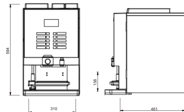
VOORAANZICHT
